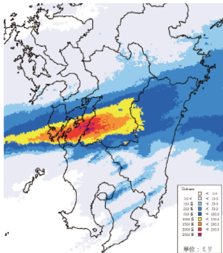
図-1.7.6 大雨特別警報発表直後の3時間雨量(7月4日午前5時) 8)
